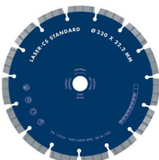
REZNA PLOČA ZA CEMENT STANDARD
